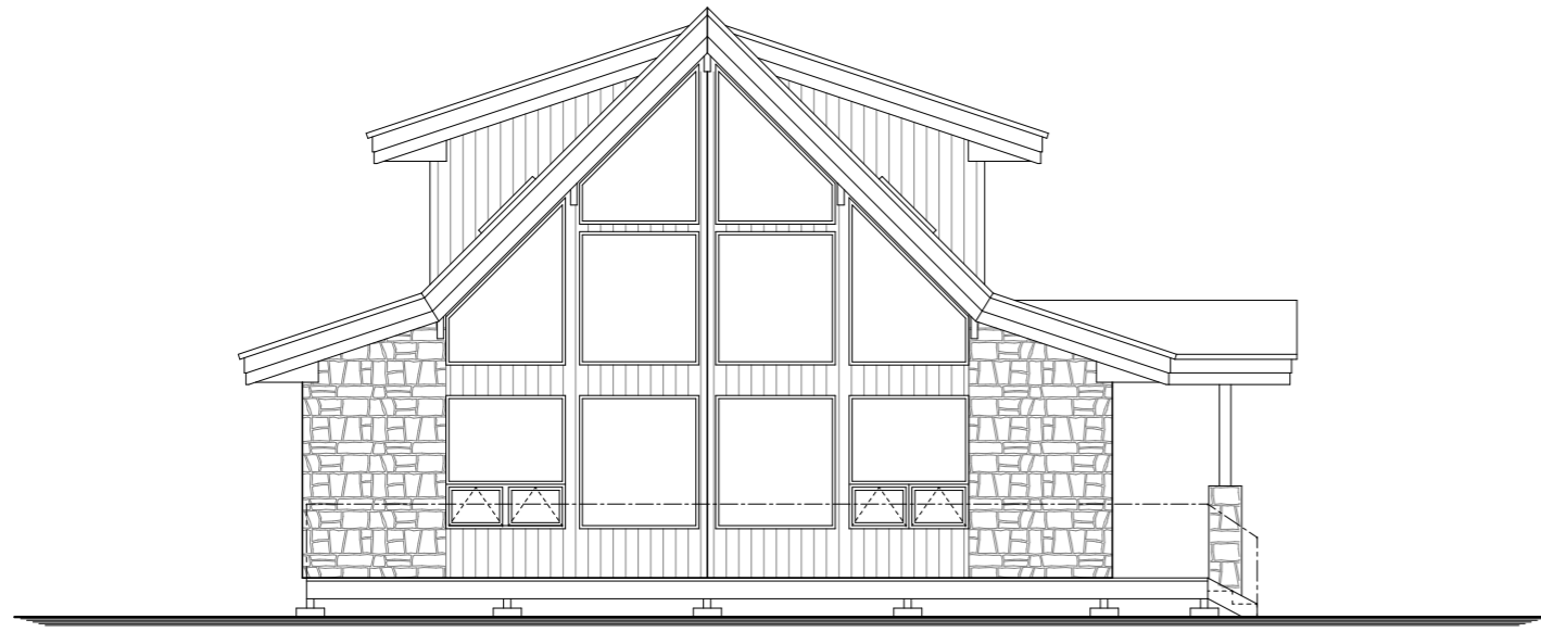
西立面图 S=1/200
