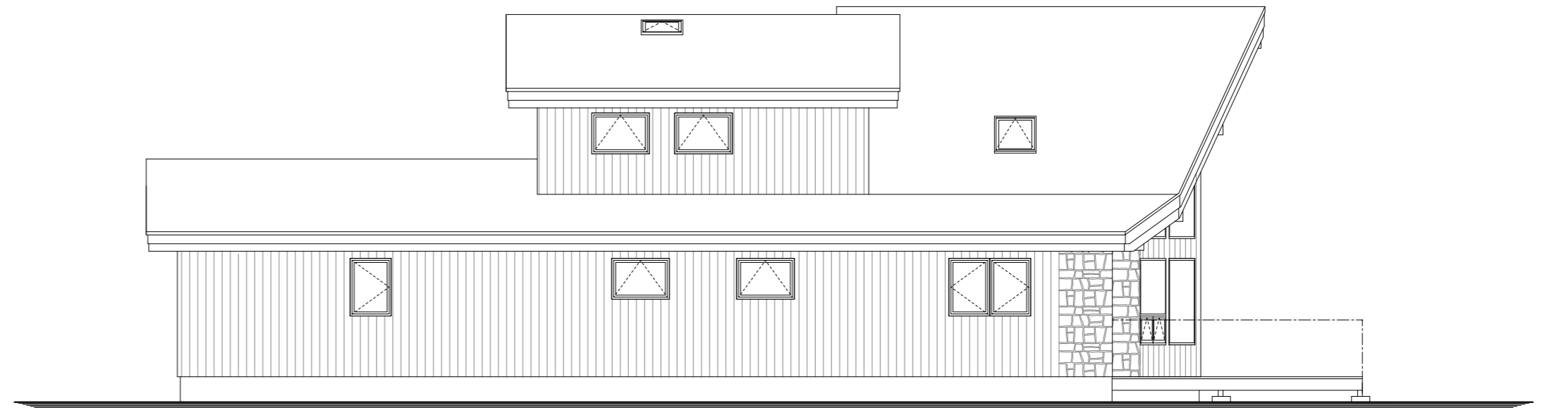
北立面图 S=1/200
