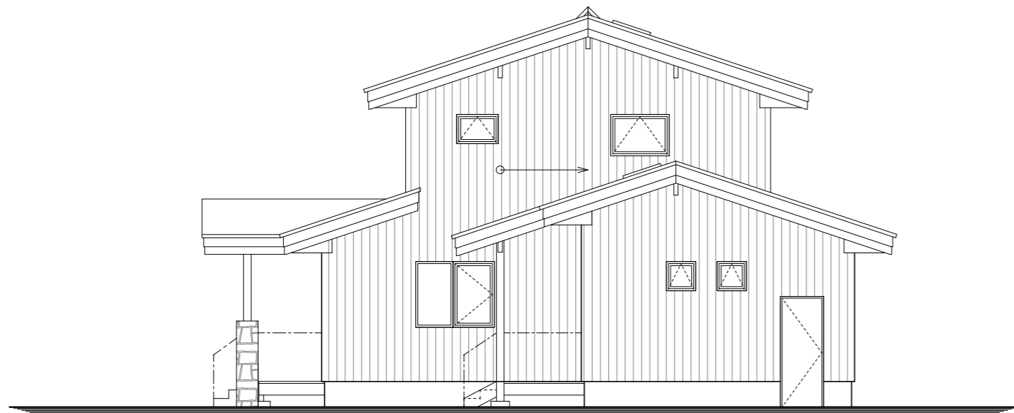
東立面图 S=1/200
